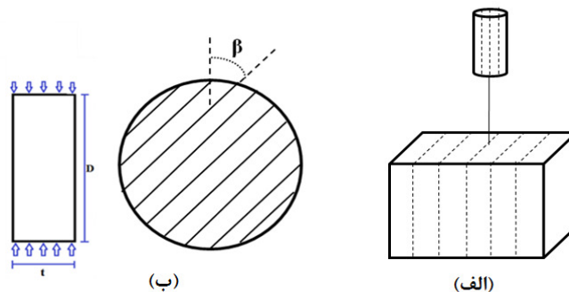
شکل ۲. (الف) مغزه‌گیری از بلوک در جهت ناهمسانگردی، (ب) نمونه دیسکی شکل تهیه شده برای آزمایش برزیلی ( \beta زاویه ناهمسانگردی، t ضخامت نمونه دیسکی شکل و D قطر نمونه دیسکی شکل که ۵۴ میلی‌متر است).
