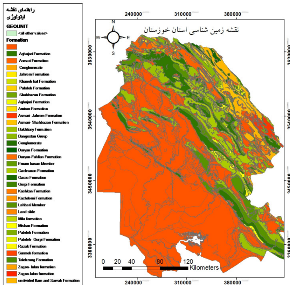
شکل ۲. نقشه زمین‌شناسی استان خوزستان
