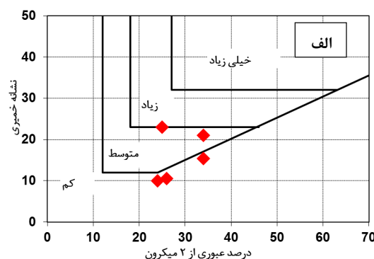
شکل ۷. ارزیابی پتانسیل تورم نمونه‌ها براساس، الف) طبقه بندی واندرو (۱۹۶۴) و ب) طبقه بندی سید و همکاران (۱۹۶۵)
