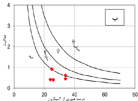
شکل ۷. ارزیابی پتانسیل تورم نمونه‌ها براساس، الف) طبقه بندی واندرو (۱۹۶۴) و ب) طبقه بندی سید و همکاران (۱۹۶۵)
