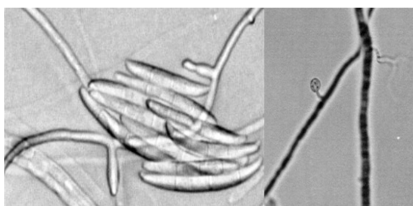
شکل ۱: مشخصات مونوفیالید و میکروکنیدی روی آن (راست) و ماکروکنیدی (چپ) F. oxysporum f.sp. lycopersici
