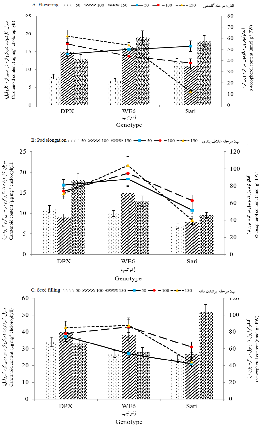
شکل ۴: میزان کاروتنوئید (نمودار ستونی) و میزان آلفاتوکوفرول (نمودار خطی) تحت شرایط تنش خشکی در ژنوتیپ‌های سویا طی مراحل رشد. میزان خطای معیار (n=4) به صورت میله‌ای نشان داده شده است
