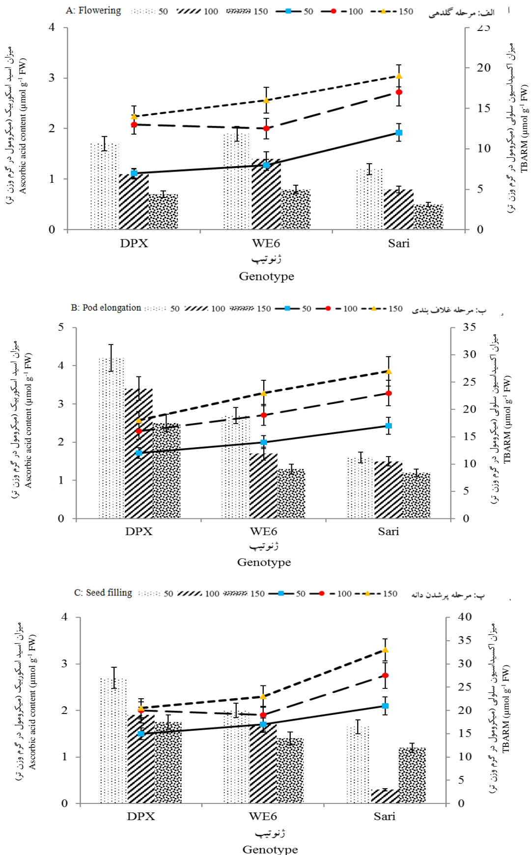
شکل ۳: میزان اسید اسکوربیک (نمودار ستونی) و مقدار شاخص اکسیداسیون سلولی (نمودار خطی) تحت شرایط تنش خشکی در ژنوتیپ‌های سویا طی مراحل رشد. میزان خطای معیار (n=4) به صورت میله‌ای نشان داده شده است
