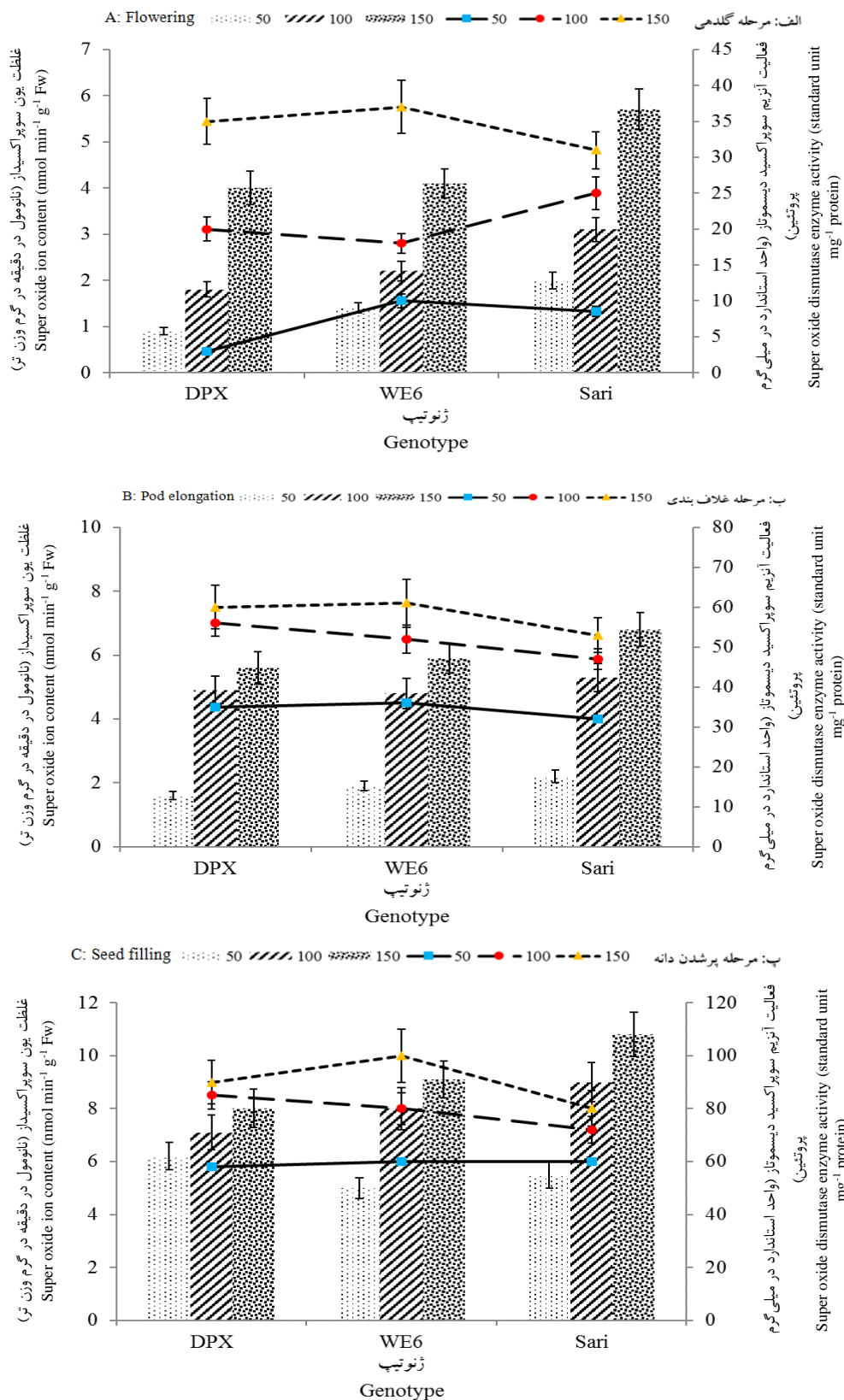
شکل ۱: میزان رادیکال سوپراکسید (نمودار ستونی) و فعالیت آنزیم سوپراکسید دیسموتاز (نمودار خطی) تحت شرایط تنش خشکی در ژنوتیپ‌های سویا طی مراحل رشد. میزان خطای معیار (n=4) به صورت میله‌ای نشان داده شده است Fig. 1: Super oxide radical content (columns) and super oxide enzyme activity (lines) during growth stages in soybean genotypes under drought stress conditions. Standard error is shown by bar sign (n=4)
