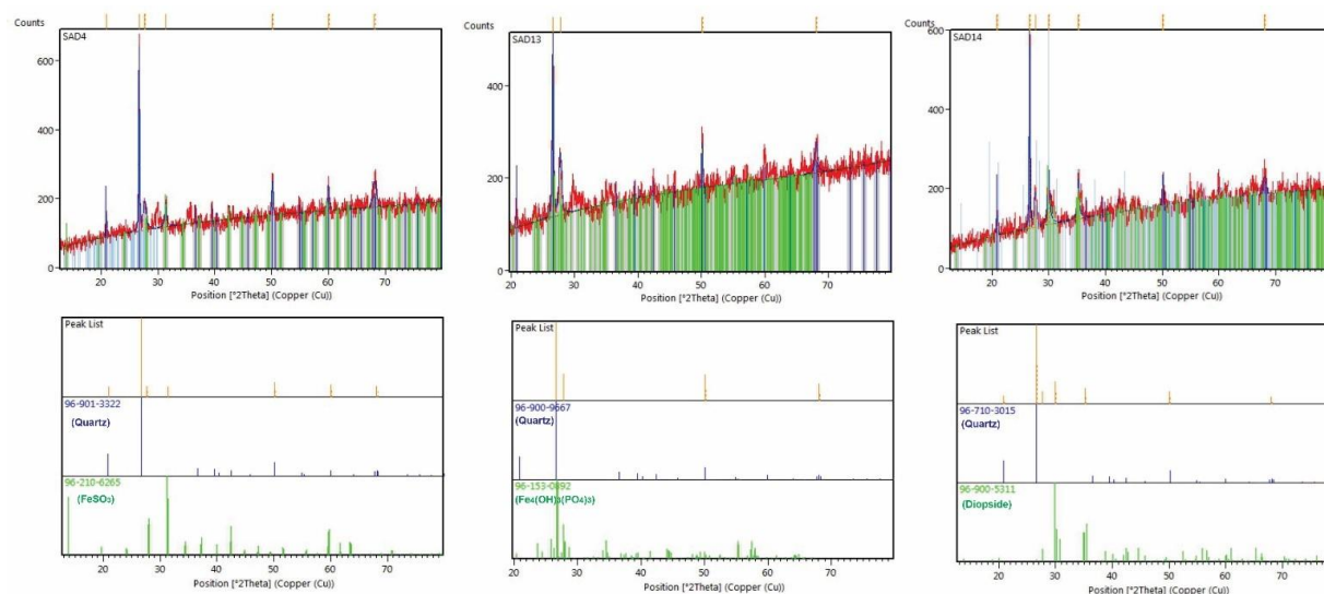
شکل ۴. الگوی پراش ایکس مربوط به سه نمونه سفالی محوطه باستانی کهنک
