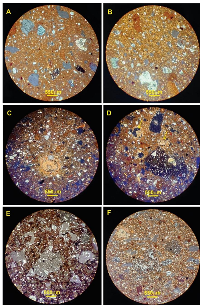
شکل ۹. تصاویر میکروسکوپی از فراوانی و تنوع فضاهای خالی در سفال‌های محوطه کهنک (نور XPL)، (A) روزن‌ها یا منافذ نامنتظم غیریکنواخت با اندازه درشت تا متوسط، (B) روزن‌ها یا منافذ نامنتظم غیریکنواخت با اندازه درشت تا متوسط، (C) حفرات نامنتظم یا روزن‌های تقریباً یکنواخت با اندازه متوسط، (D) پرشدگی منافذ سفال به صورت کامل و جزئی توسط بلورهای کلسیت که احتمالاً در طی دفن نمونه انجام شده است، (E و F) درصد فراوانی بالای فضاهای خالی در برخی نمونه‌های مورد مطالعه.
