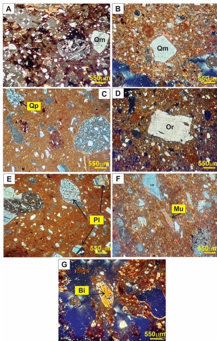
شکل ۶. تصاویر میکروسکوپی (XPL) از انواع انکلوژیون‌های تشکیل‌دهنده سفالینه‌های مورد مطالعه، A) کوارتز تک بلور پلوتونیک (Qm)، B) کوارتز تک بلور ولکانیک (Qm)، C) کوارتز چند بلور دگرگونی تبلور مجدد (Qp)، D) فلدسپات ارتوکلاز (Or)، E) فلدسپات پلاژیوکلاز (Pl)، F) میکای مسکویت (Mu) و G) میکای بیوتیت (Bi).
