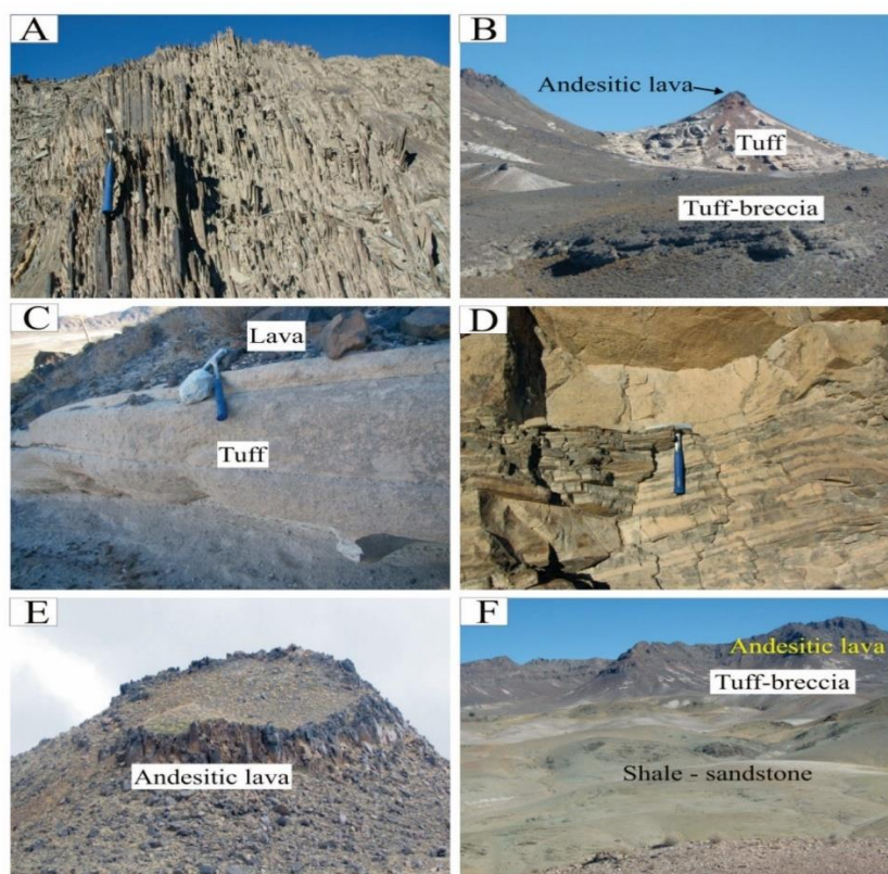
شکل ۱۵. A) نمایی از شیل و ماسه‌سنگ‌های دگرگون‌شده در جنوب‌شرق سربیشه، دید به‌سوی شمال‌غرب، B و C) حضور گدازه‌های آندزیتی بر روی توف‌ها در جنوب‌شرق سربیشه، دید به‌سوی شمال‌شرق، D) لیتیک توف دربرگیرنده شیشه آتشفشانی و دارای حالت نواری در جنوب‌شرق سربیشه، E) رخنمون واحدهای گدازه‌ای آندزیتی در بخش‌های مرکزی و شمال‌شرق سلم‌آباد به‌صورت گنبدیهایی با ساخت توده‌ای و گاهی ستونی، دید به‌سوی شمال-شرق، F) نمایی از قرارگیری گدازه و آذرآواری‌ها بر روی شیل و ماسه‌سنگ در شرق روستای کهنک، دید به‌سوی شمال‌شرق (گودرزی و همکاران، ۱۳۹۳). Fig. 15. A) View metamorphosed shale and sandstone in southeast of Sarbisheh, look toward northwest, B and C) Presence of andesitic lavas on top of tuffs in southeast of Sarbisheh, look toward northeast, D) Lithic tuff with volcanic glass and band shape in southeast of Sarbisheh, E) Outcrops of andesitic units in central and northeastern parts of Salm abad as domes with massive and columnar structure, look toward northeast, F) View of lava and pyroclastics on top of shale and sandstone in east of Kahnek village, view toward northeast (Goodarzi et al., 2015).
