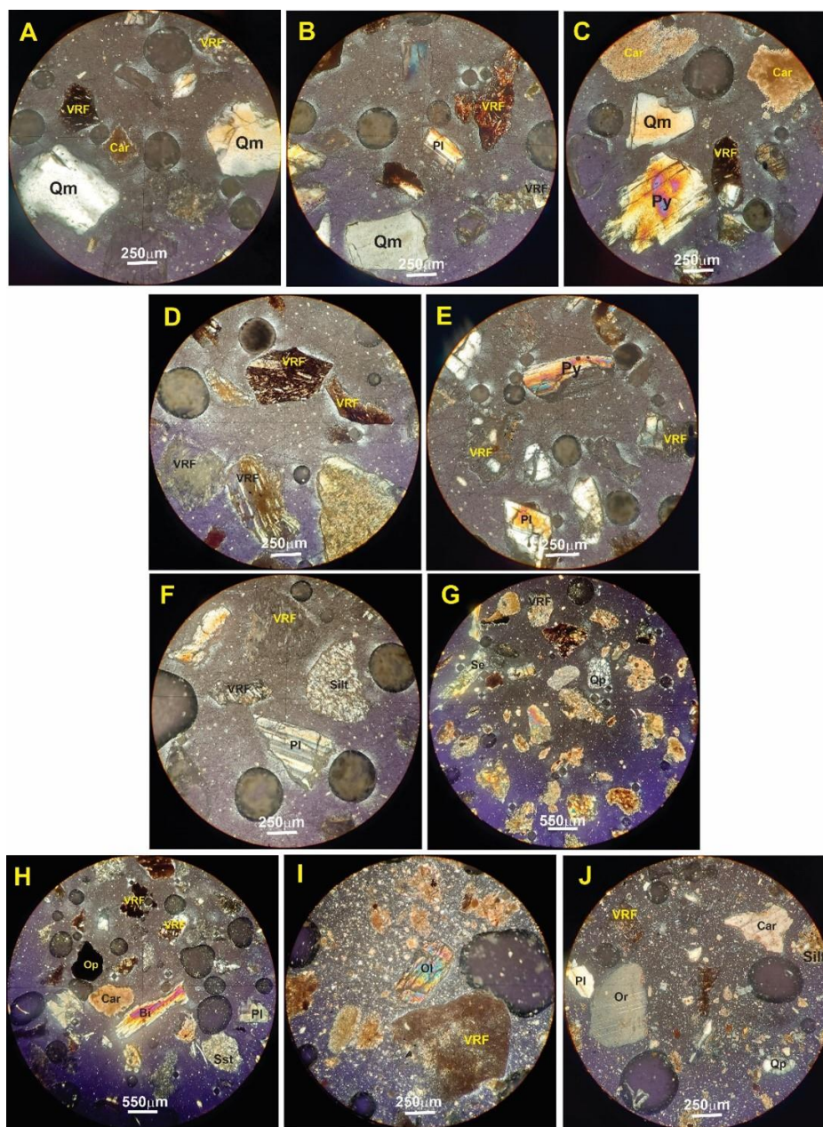
شکل ۱۳. تصاویر میکروسکوپی (XPL) از اجزاء تشکیل‌دهنده نمونه‌های رسوب رودخانه مجاور محوطه کهنک، این قطعات شامل کوارتز تک‌بلور (Qm)، کوارتز چندبلور (Qp)، پلاژیوکلاز (Pl)، ارتوکلاز (Or)، قطعات الیون (Ol)، پیروکسن (Py)، خرده‌سنگ‌های ولکانیکی (VRF) و آذرین سرپانتینی شده (Se)، خرده‌سنگ‌های رسوبی ماسه‌سنگی (Sst)، سیلتستونی (Silt) و کربناته (Car)، بیوتیت (Bi) و کانی‌های سنگین تیره (Op).
