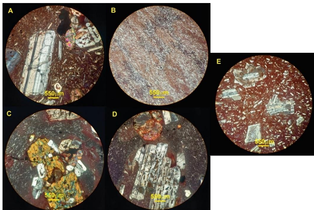
شکل ۱۲. تصاویر میکروسکوپی (XPL) قطعات گراولی پراکنده در اطراف محوطه و دیواره کانال رودخانه مجاور محوطه. (A) آندزیت بازالتی، (B) بازال، (C) پیروکسن آندزیت با بافت گلومروپورفیری همراه با پلاژیوکلازهای با بافت غربالی، (D) آندزیت با پلاژیوکلازهای با بافت غربالی، (E) آندزیت.
