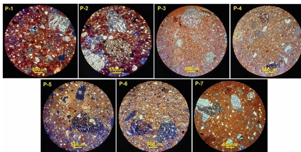
شکل ۳. تصاویر میکروسکوپی سفالینه‌های محوطه کهنک (نور XPL) که اجزاء تشکیل‌دهنده خمیره‌ی آن‌ها، به ویژه ماتریکس رسی در رنگ‌های مختلف قابل مشاهده است.
