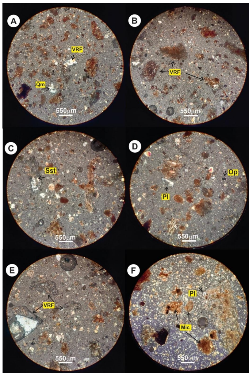
شکل ۱۰. تصاویر میکروسکوپی (نور XPL) از اجزاء تشکیل‌دهنده نمونه‌های خاک سطحی محوطه کهنک. کوارتز تک‌بلور (Qm)، کوارتز چندبلور (Qp)، پلاژیوکلاز (Pl) خرده‌سنگ‌های ولکانیکی حدواسط و مافیک (VRF)، خرده‌سنگ رسوبی ماسه‌سنگی (Sst) و قطعات میکریتی کربناته (Mic) در تصاویر مشخص شده است.
