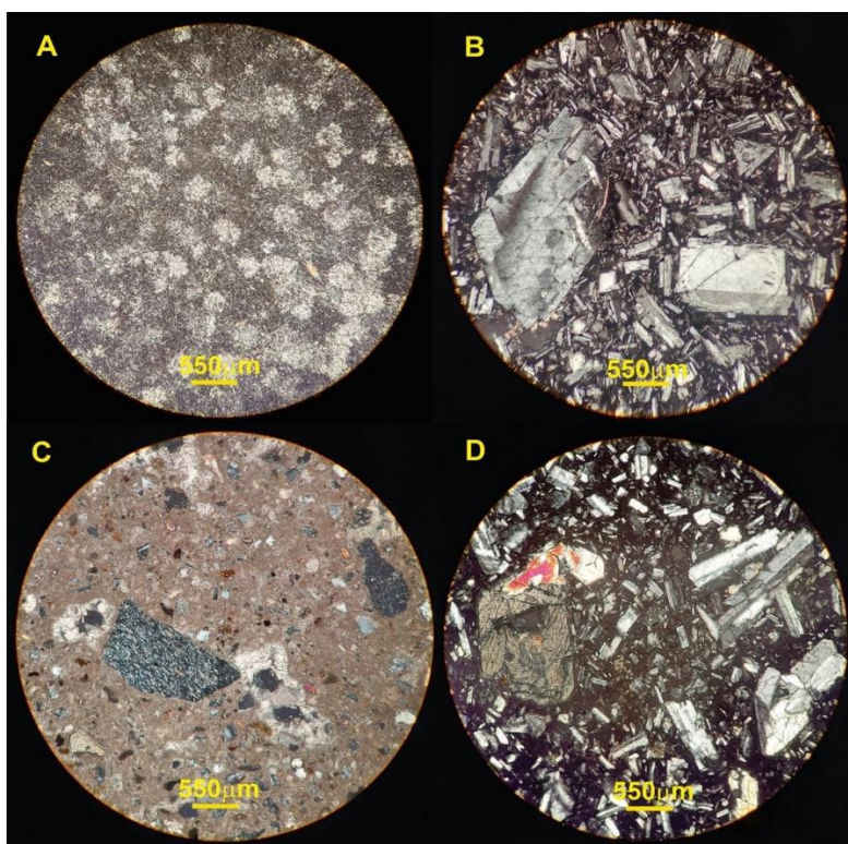
شکل ۱۱. تصاویر میکروسکوپی (XPL) قطعات گراولی پراکنده در اطراف محوطه و دیواره کانال رودخانه مجاور محوطه. (A) سنگ ولکانیکی دگرسان شده (احتمالاً شیشه آتشفشانی)، (B) آندزیت، (C) آهک ماسه‌ای همراه با خرده‌سنگ‌های ولکانیکی و دگرگونی، (D) آندزیت.
